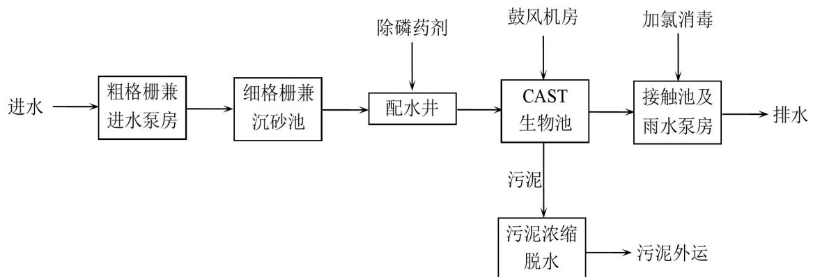
图 3 仙林污水处理厂污水处理工艺流程图
