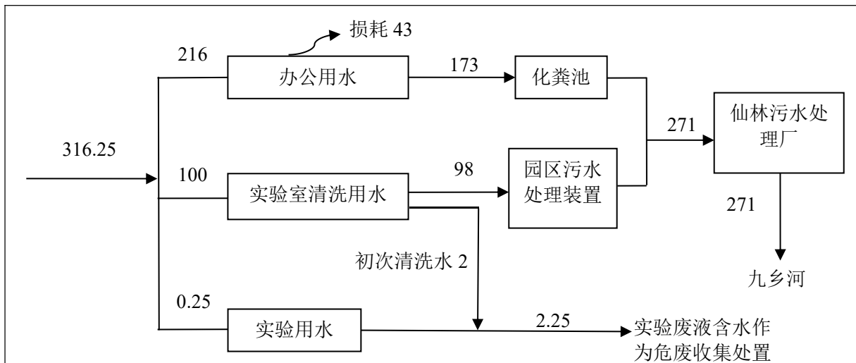
图 6-1 建设项目用水平衡图 (t/a)
