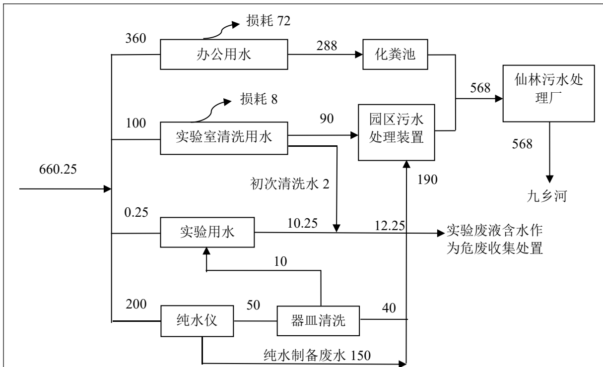
图 6-2 建设项目用水平衡图 (t/a)
