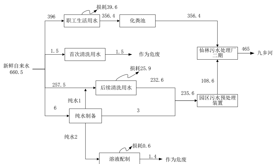
图 6-3 建设项目水平衡图 (t/a)
