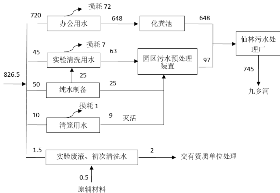
图 4-2 建设项目水平衡图 (t/a)
