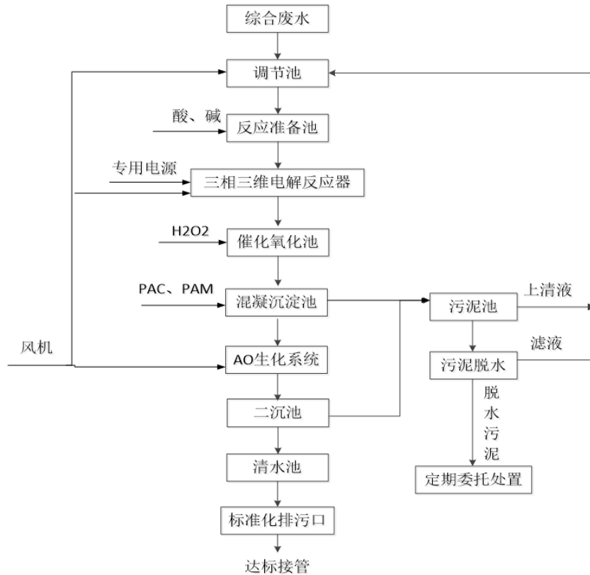
图 4-3 建设项目废水预处理工艺流程图
