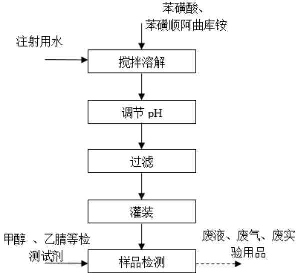
图 2-1 苯磺顺阿曲库铵研发工艺流程
