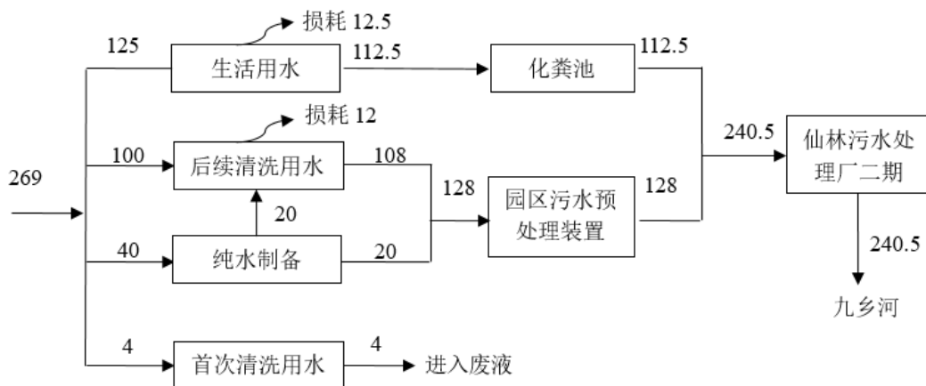
图 4-2 建设项目水平衡图 (t/a)
