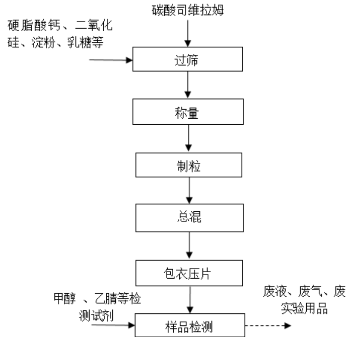
图 2-2 碳酸司维拉姆片研发工艺流程
